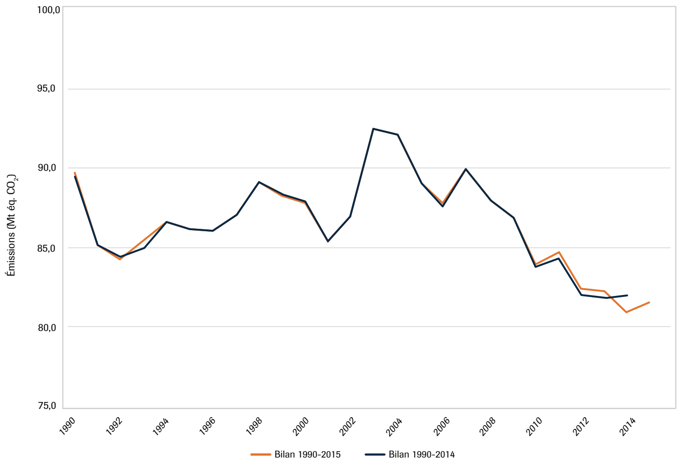
Figure 3. Comparaison des inventaires québécois de GES 1990-2014 et 1990-2015
