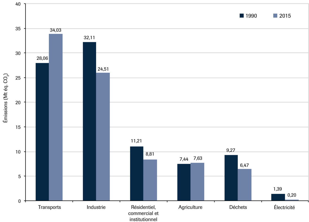
Figure 6. Émissions de GES au Québec par secteurs d'activité en 1990 et 2015
