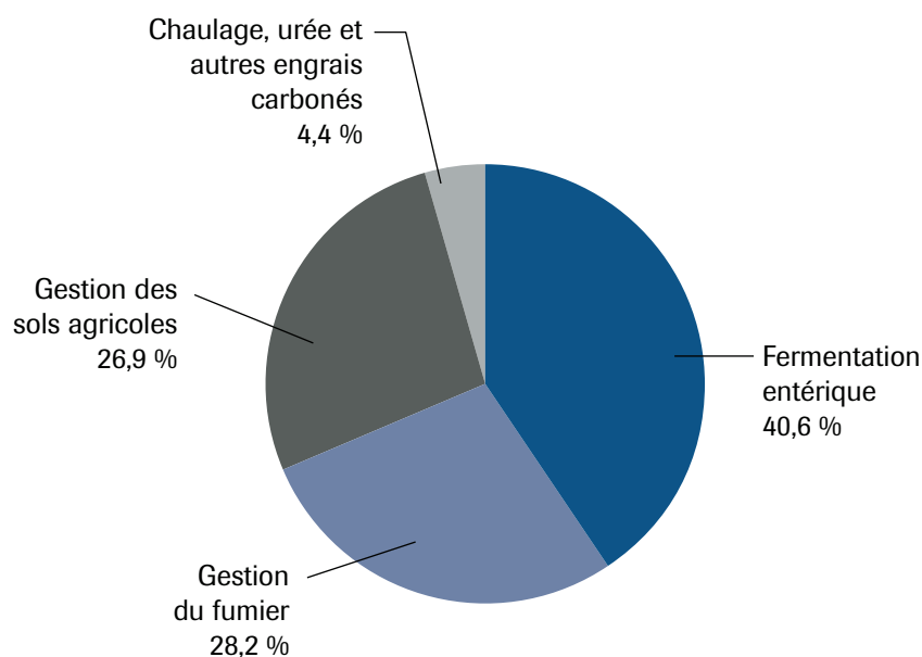
Figure 13. Répartition des émissions de l'agriculture
