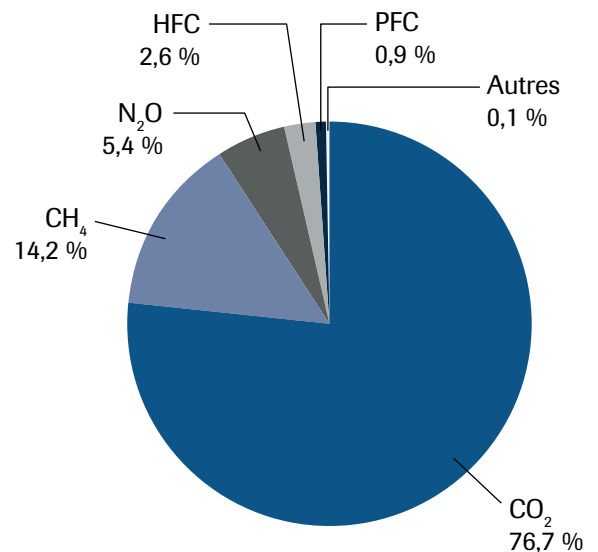
Figure 2. Répartition des émissions de GES au Québec, en 2015, selon le type de gaz
