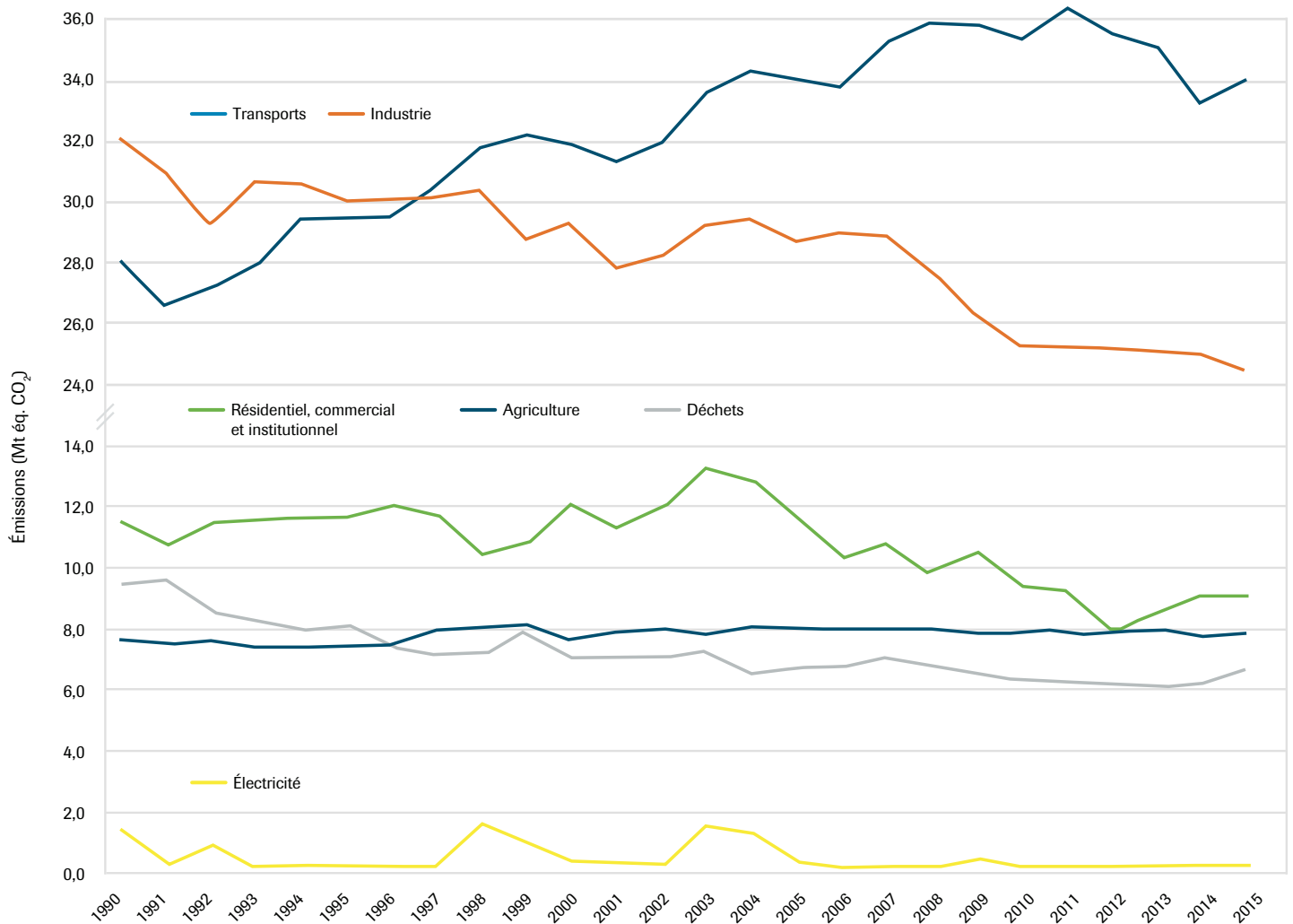
Figure 5. Émissions de GES au Québec par secteurs d'activité entre 1990 et 2015
