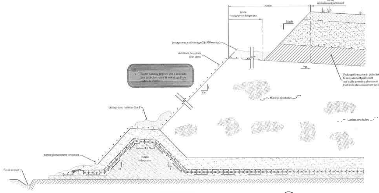
COUPE TYPE INSTALLATION DU RECROUVREMENT TEMPORAIRE ÉCHELLE AUCUNE
