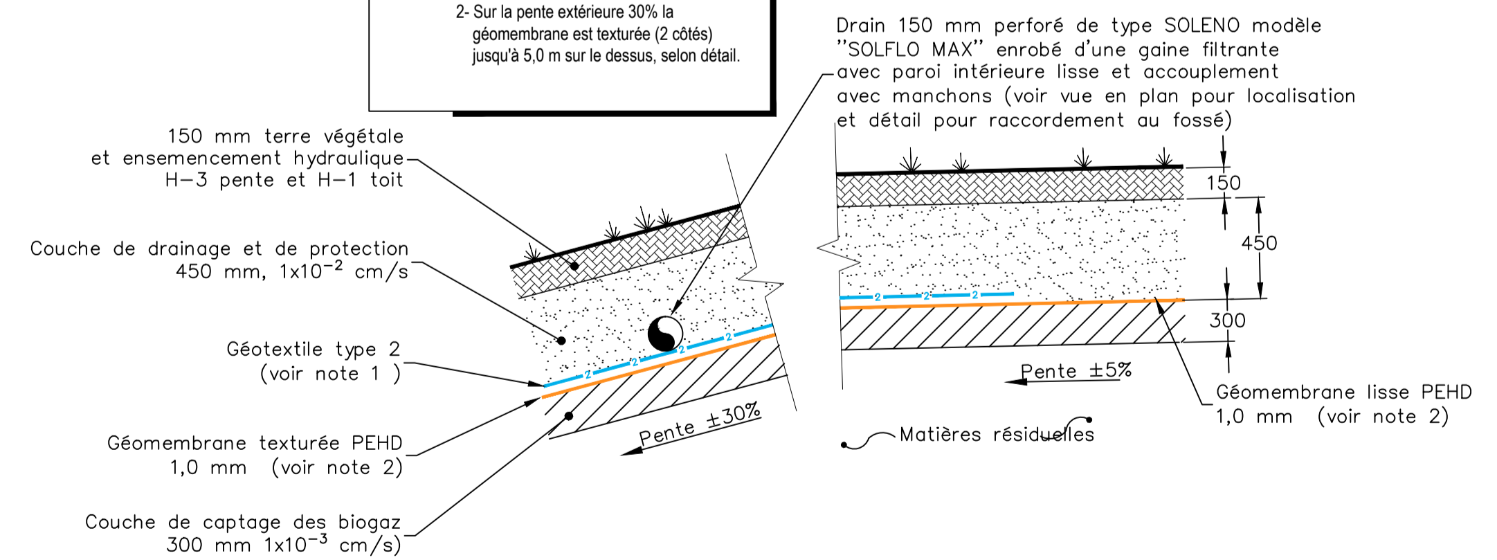
DÉTAIL TYPE : RECOUVREMENT FINAL ECH.: AUCUNE
