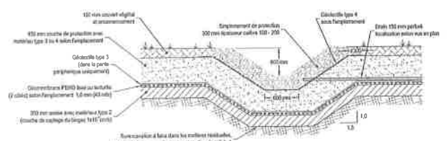
DÉTAIL TYPE FOSSE ÉCHELLE AUCUNE
