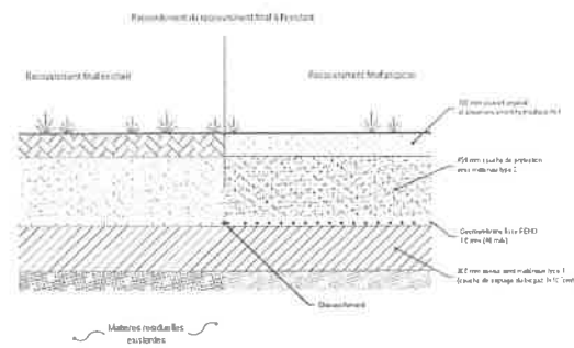
DÉTAIL TYPE - RECROUVREMENT PERMANENT RACCORDEMENT À L'EXISTANT ÉCHELLE AUCUNE
