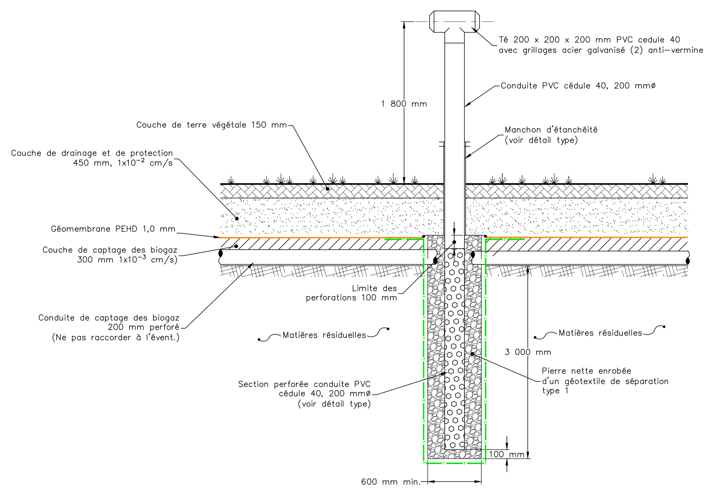
DÉTAIL TYPE : PUIS PASSIF DE CAPTAGE ET D'ÉVACUATION DES BIOGAZ ECH.: AUCUNE
