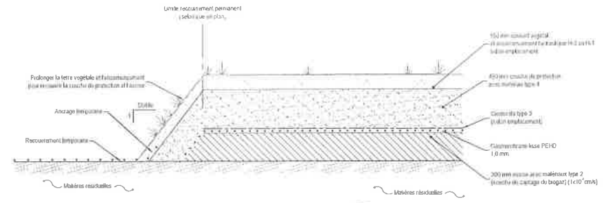
DÉTAIL-TYPE 16 LIMITE DU RECOUVERTEMENT FINAL ÉCHELLE: NATURELLE
