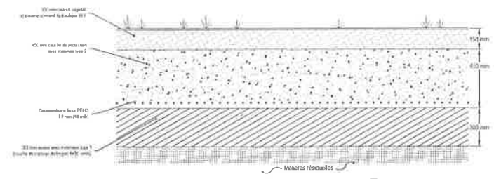
DÉTAIL TYPE RECROUVREMENT FINAL ÉCHELLE AUCUNE
