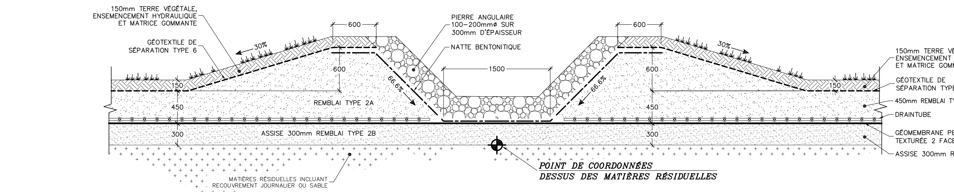
DÉTAIL TIPIQUE DESCENTE PLUVIALE Echelle: Aucune
