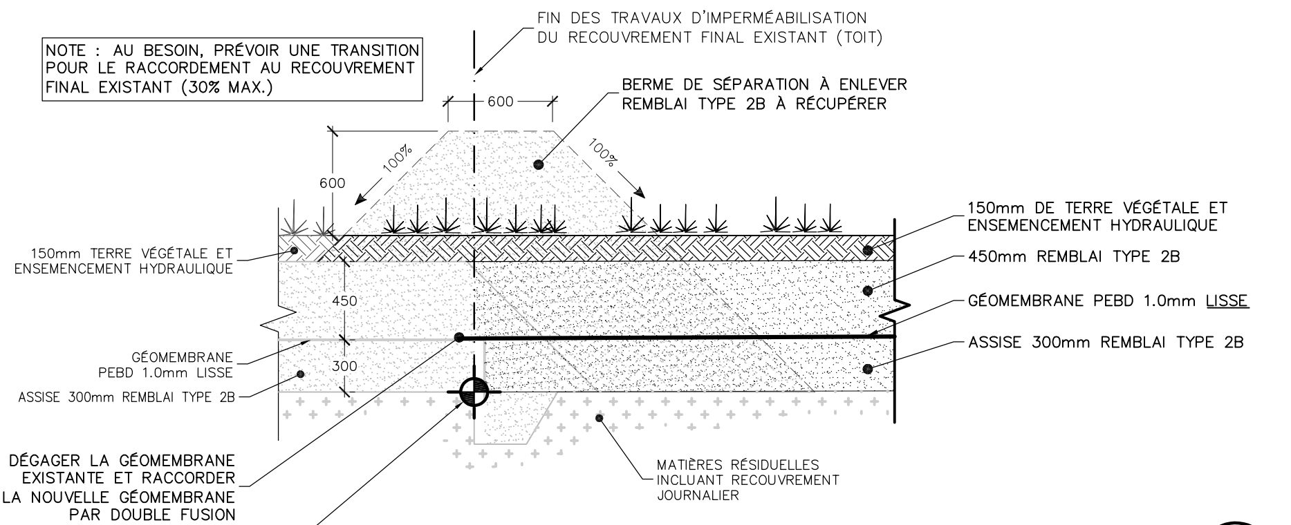
DÉTAIL TIPIQUE RACCORDEMENT DU SYSTÈME D'IMPERMÉABILISATION DU RECouvreMENT FINAL À L'EXISTANT Echelle: Aucune
