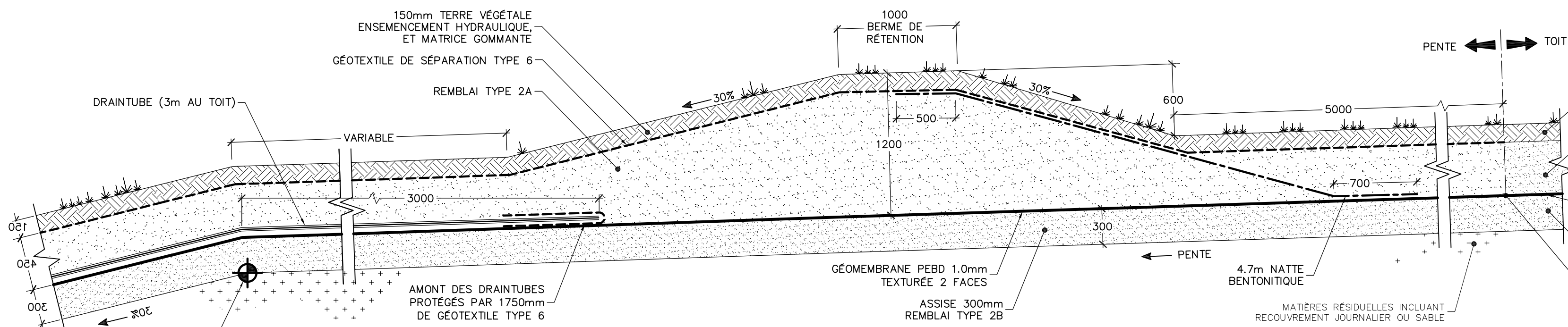
DÉTAIL TIPIQUE RECouvreMENT FINAL BERME DE RÉTENTION HAUT DE TALUS Echelle: Aucune
