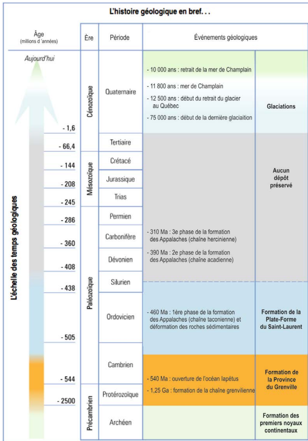
Figure 3.2 : Histoire géologique
