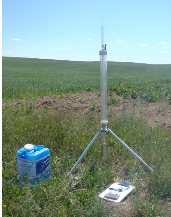
Figure 3.12 : Réalisation d'un essai au perméamètre de Guelph à Trois-Pistoles en juillet 2014.
