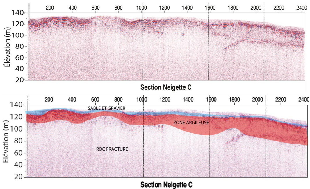
Figure 3.3 : Exemple de résultat et d'interprétation d'un levé sismique de la vallée de la rivière Neigette à Saint-Anaclet-de-Lessard.
