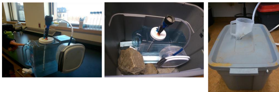
Figure 3.8. Conception des collecteurs d'eau de pluie utilisés dans le PACES-NEBSL.
