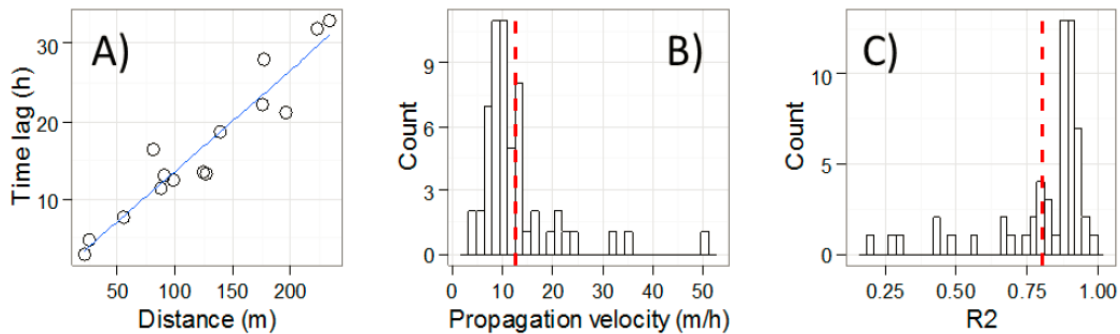
Figure 7.20. A) Temps de réponse de l'onde phréatique en fonction de la distance perpendiculaire à la berge pour un événement de crue (41). 9B) Histogramme de la répartition des 57 événements en fonction de la vitesse de propagation de l'onde phréatique. 9C) Histogramme des coefficients de régression de la relation linéaire entre le temps de réponse des piézomètres et la distance perpendiculaire à la berge (Buffin-Bélanger et al. en révision).
